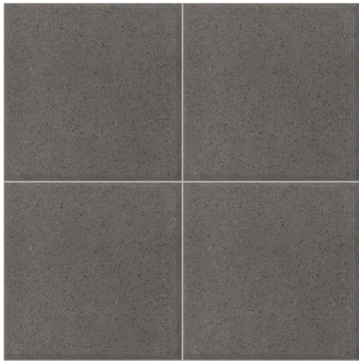
Code: VG15-ECO-G-60 Màu sắc: Xám đá bụi Dimension: 150x150x60mm
